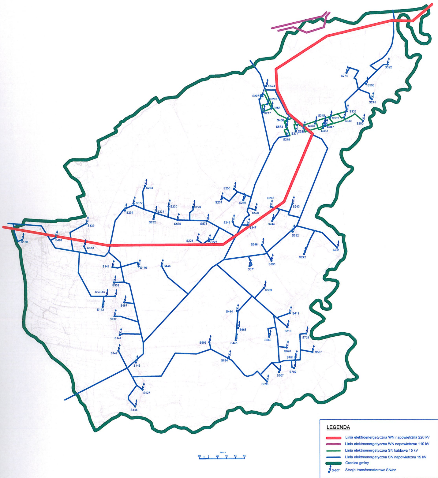
Rysunek I. Mapa systemu elektroenergetycznego na terenie Gminy Miedźna
